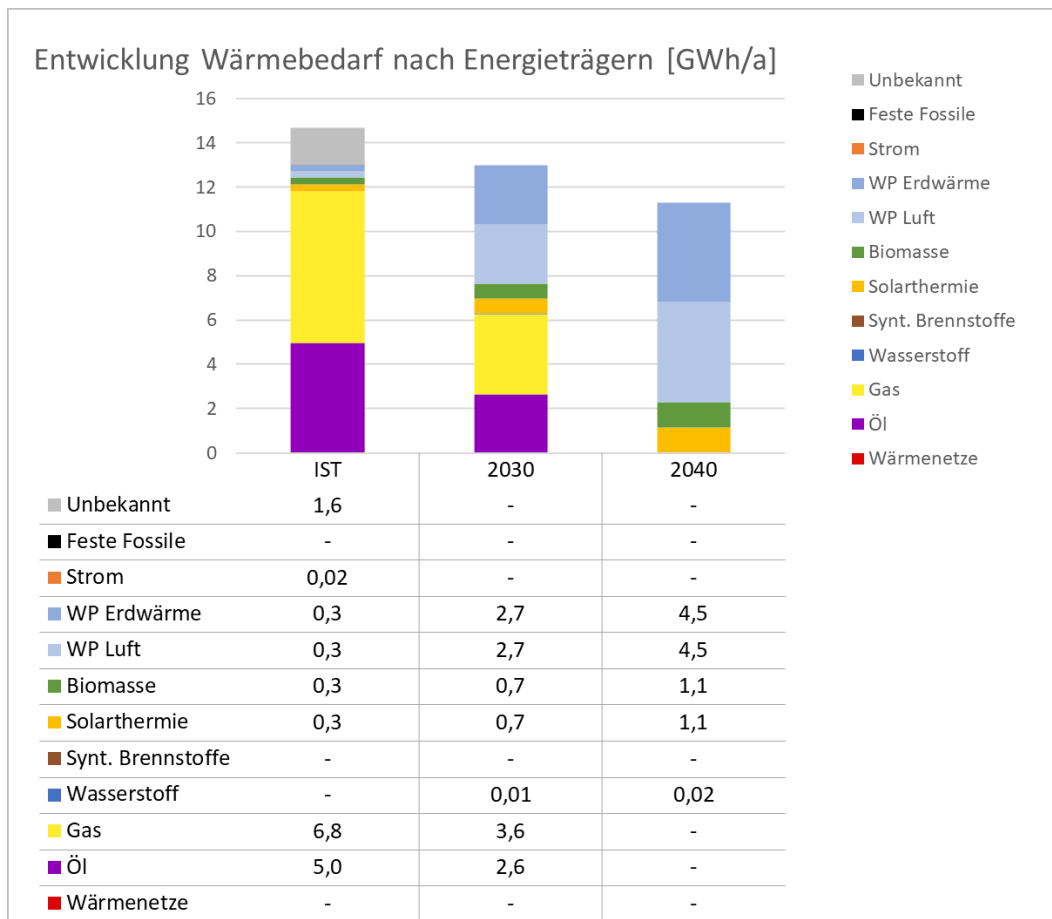
Abbildung 14: Entwicklung des Wärmebedarfs und eingesetzte Energieträger in Rümmingen: IST, 2030, 2040. Die angesetzten Reduktionsfaktoren sind im vorigen Kapitel erläutert.
