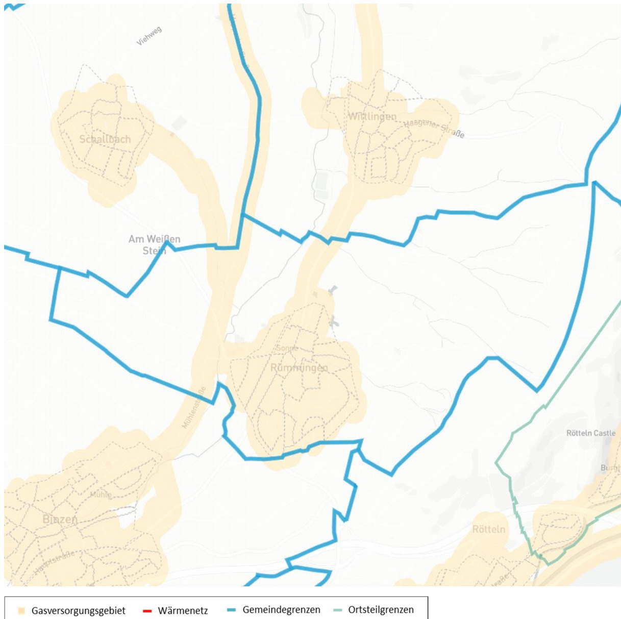
Abbildung 6: Vorhandene Wärme-Infrastruktur in Rümmingen.
